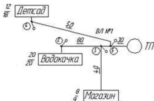
Рисунок - Расчётная схема ВЛ 0,38/0,22 кВ
