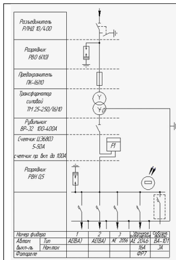
Рисунок - схема однолинейная электрическая КТП-89У1 25-250/6-10/0,4 У1
