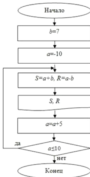
Рис. 1. ... алгоритм
