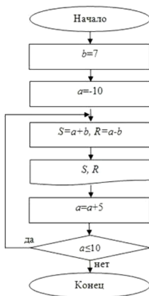
Рис. 1. ... алгоритм
